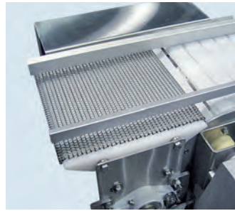
Приводной мостик
